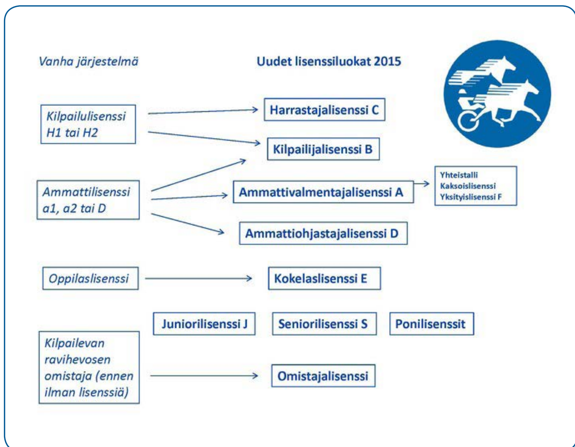
Kuva 1: Raviurheilun lisenssijärjestelmä.
